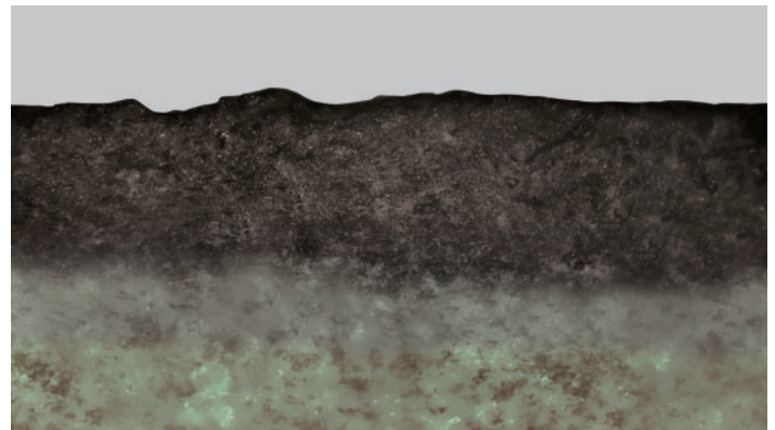
Schnitt durch ein Nadura-Element mit extrem verstärkter Nutzschrift, direkt aufgebracht auf eine Spezialplatte – im Elektronenmikroskop.
