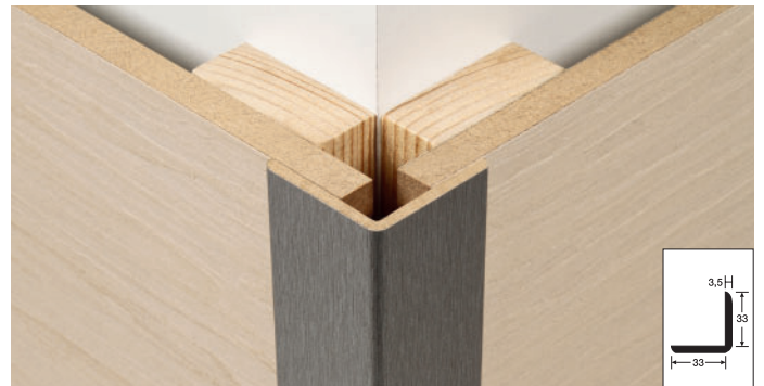
Winkelleiste groß
