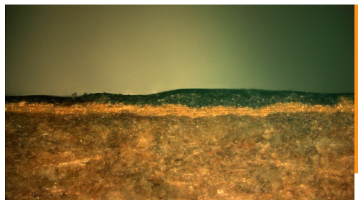
Schnitt durch Laminat mit Nutzschrift aus Overlay, Dekorpapier und HDF-Mittellage im Elektronenmikroskop.
